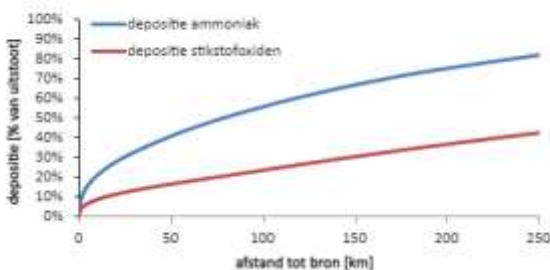
Percentage van de totale stikstofuitstoot van een bron dat binnen 250 km neerkomt
