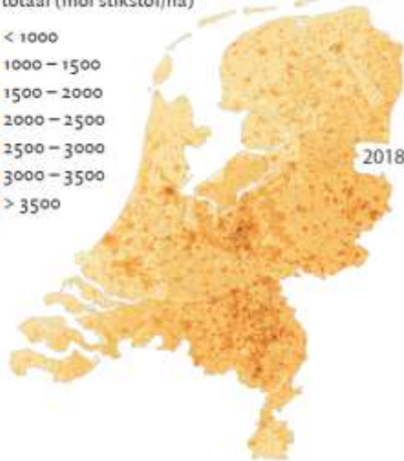
jaartotaal (mol stikstof/ha)
