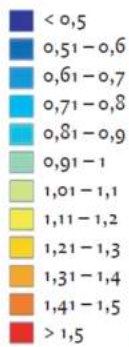
Tropomi jaargemiddelde (mg N/m 3 )
