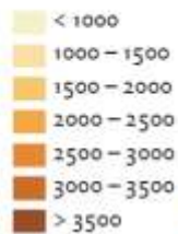
jaartotaal (mol stikstof/ha)
